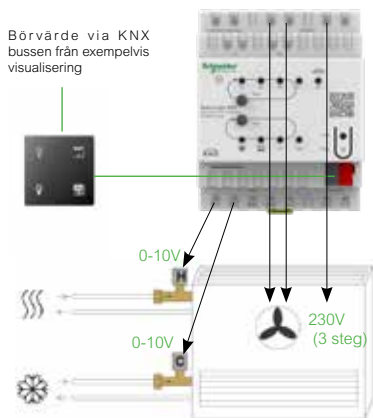
Tempregulator i aktorn, börvärde via KNX buss, fläkt 3 med steg
