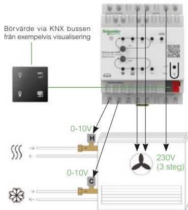
Tempregulator i aktören, börvärde via KNX buss, fläkt 3 med steg
