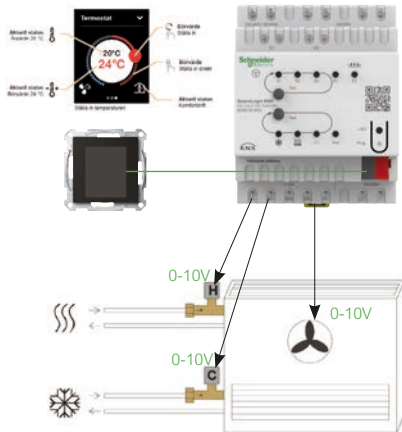
Tempregulator och börvärde i Multi Touch Pro, fläkt med 0-10V
