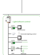
Våning 2
