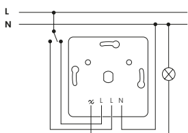
Installation med neutralledare
