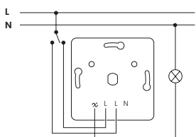
Installation utan neutralledare
