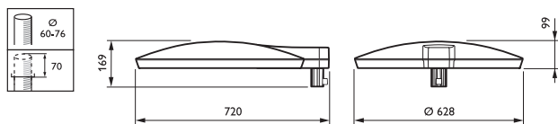
BPP531 GRN60-/830 II DM FG AL GR
